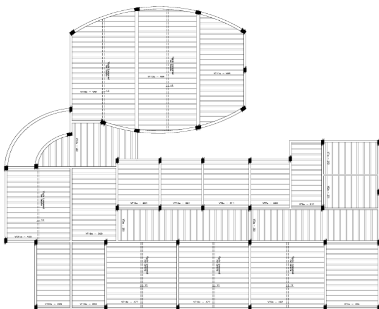
Distribuição dos Vagos Treilhados das Lajes Esc. 1:75
